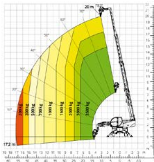
Load chart with WINCH 3,500 kg ATT - 02 - 002
