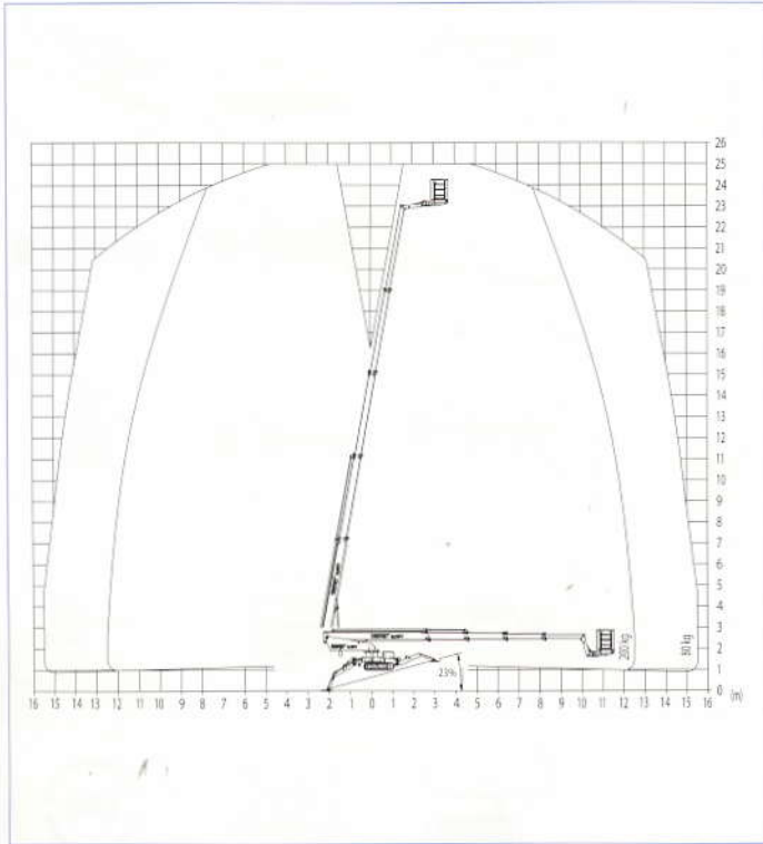
Arbeitsdiagramm
